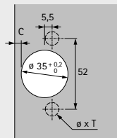
Opliggend (basis B 11,5 mm)
