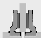
Half opliggend (basis B 3 mm)
